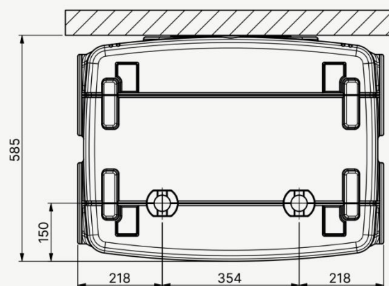
Dolní pohled
