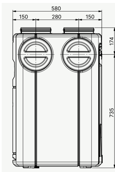
Horní pohled
